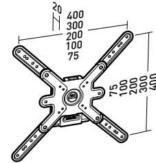
Platine écran
