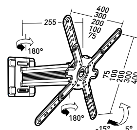
Platine écran
